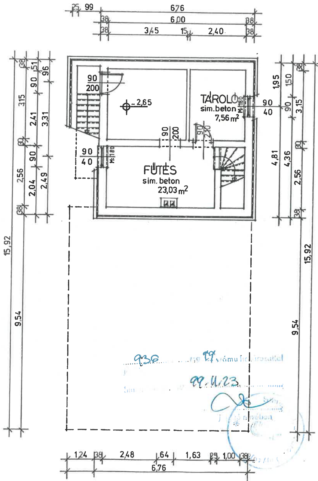
PINCESZINT ALAPRAJZ M=1:100
