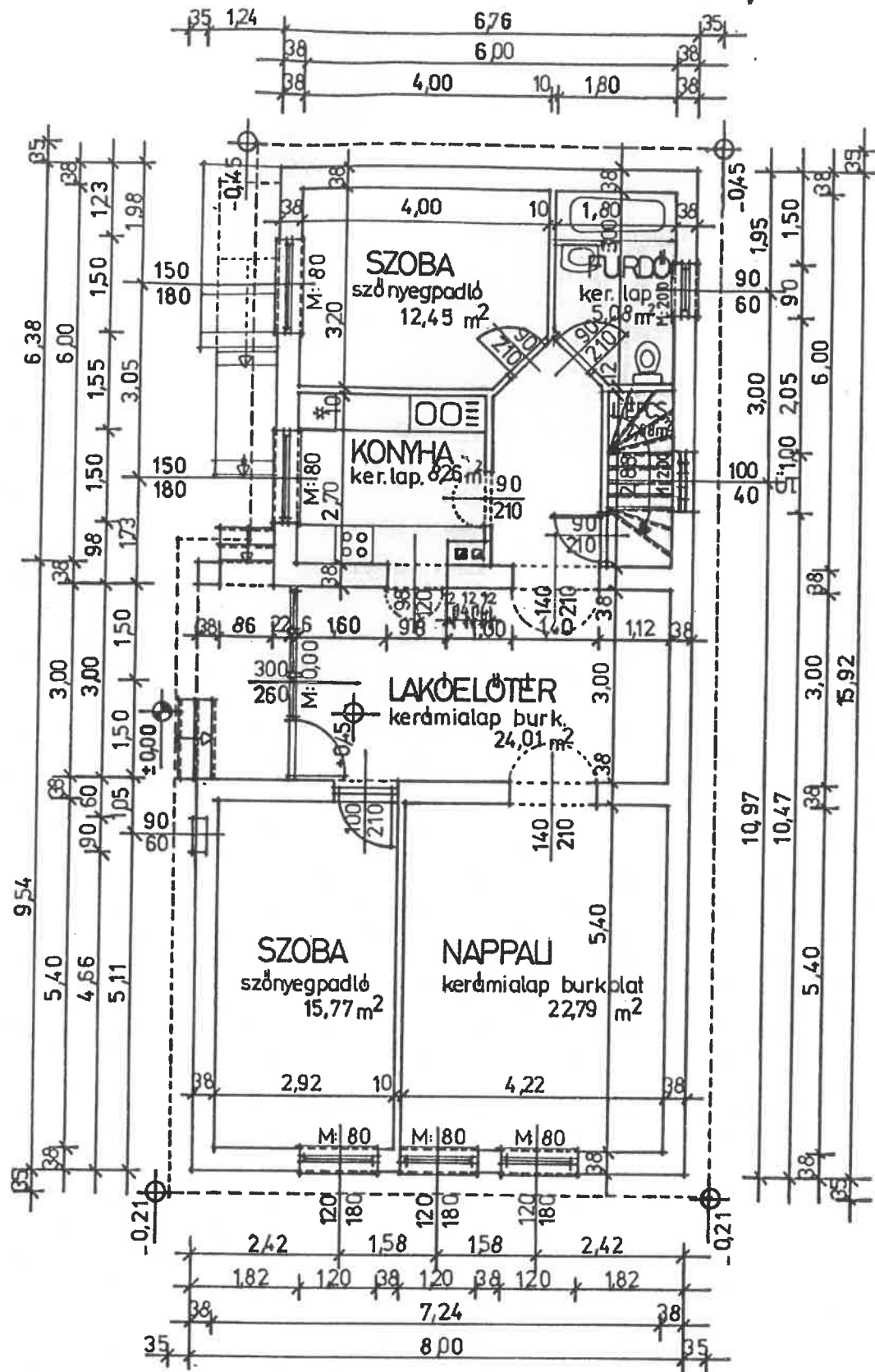
FÖLDSZINTI ALAPRAJZ M=1:100
